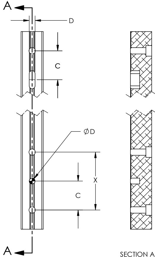
SECTION A-A
